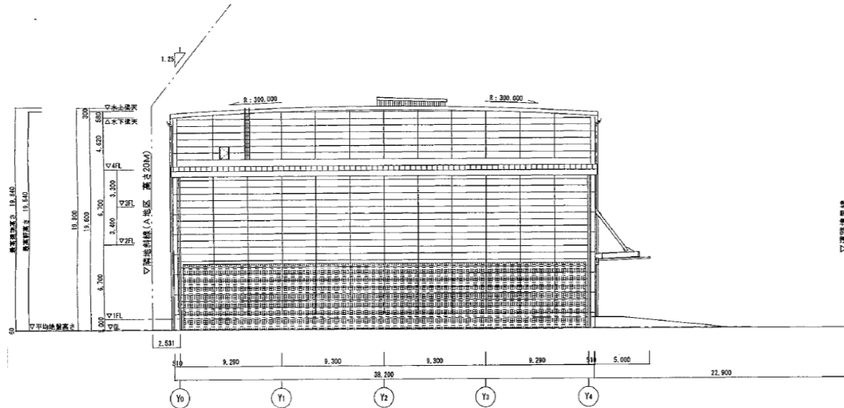
東立面図
